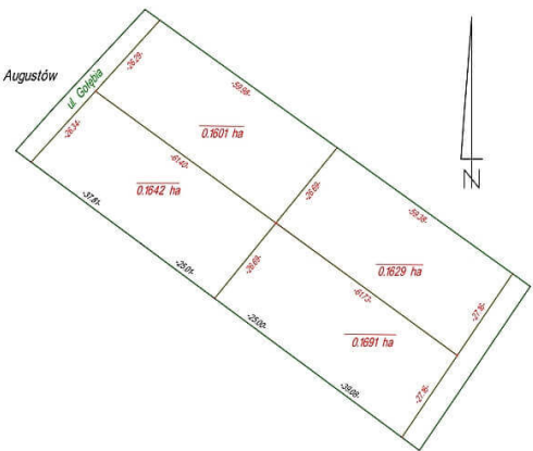
SZKIC WYZNACZENIA PROJEKTU PODZIAŁU DZIAŁKI
